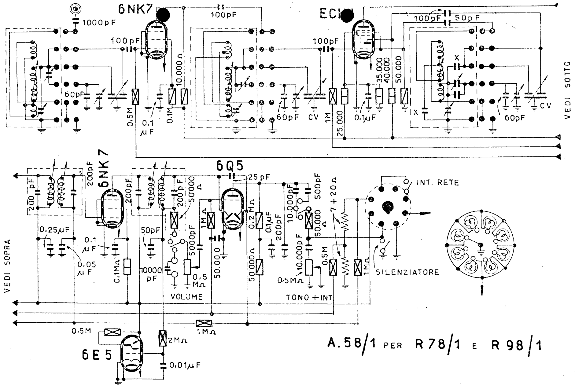
UNDA RADIO - Mod. R 78/1 e mod. R 98/1 - Schema della parte AF/MF (telaio A 58/1). Tensioni 6NK7: 200 V pl., 100 V sch.; ECH4 e 6NK7 (MF): 250 V pl., 105 V osc., 105 V sch.; 6Q7: 150 V pl., 6E5: 250 V pl. 45 V schermo. Media frequenza: 450 kc/s.
